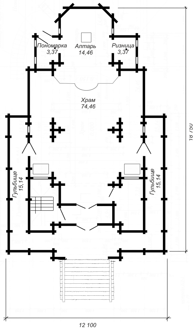
План первого этажа
